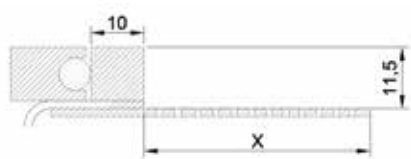
Flansza perforowana
