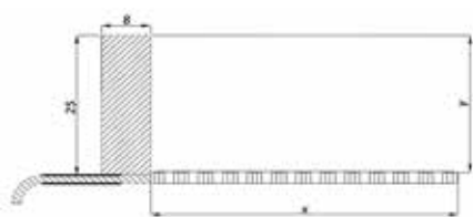
Flansa perforowana
