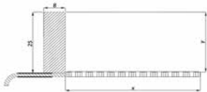
Flansa perforowana
